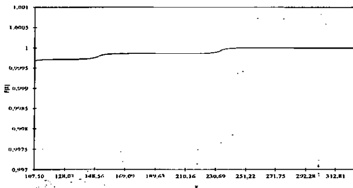
Gráfico 7. Función de distribución empírica, sobre la cola derecha, para la Empresa Completa
