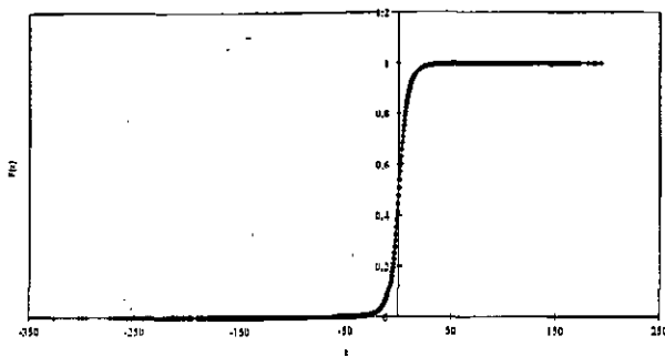
Gráfico 1. Función de distribución según convolución de los retornos conjuntos
