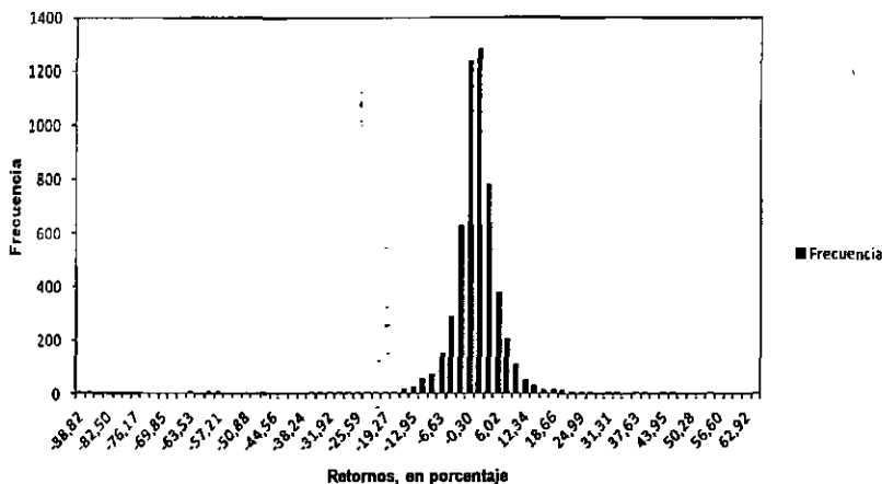
Gráfico 2. Histograma según convolución de retornos de las empresas
