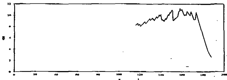
Gráfico 5. Mean ExcessLoss para la Empresa Completa
