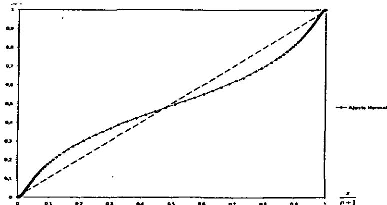
Gráfico 3. Cuantil-Cuantil, bajo supuesto de normalidad
