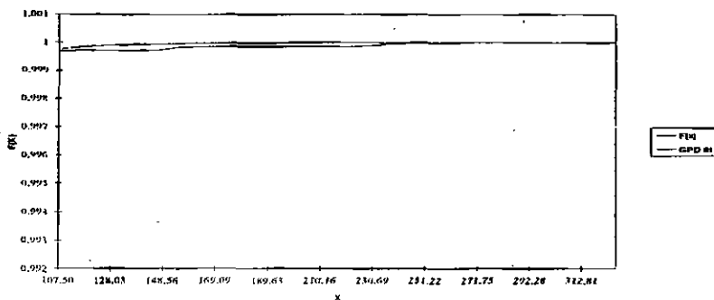
Gráfico 8. Ajuste de DGP y valores muestrales para la Empresa Completa (N=12.000 y pasos de interpolación 32.000)
